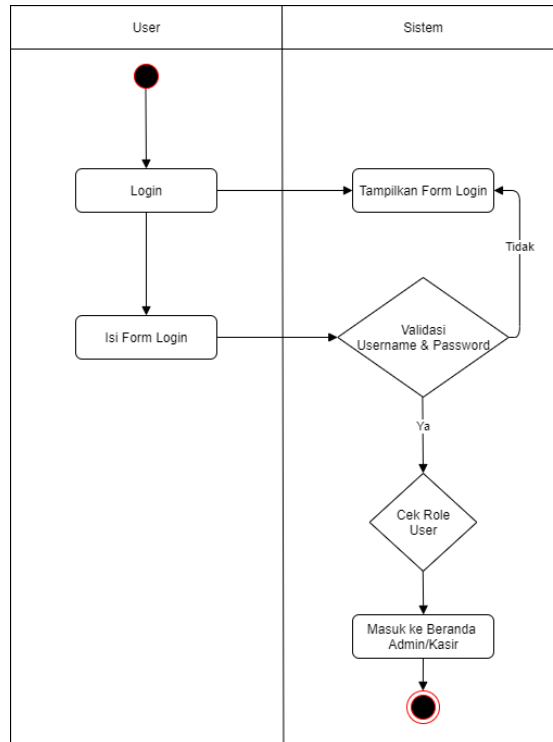
Gambar 1. Login
