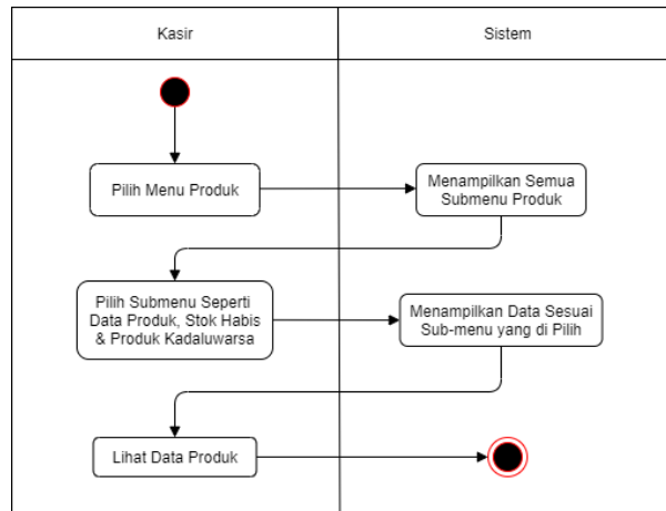
Gambar 3. Produk
