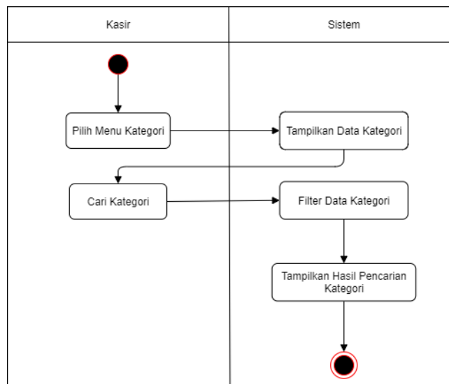
Gambar 2. Kategori
