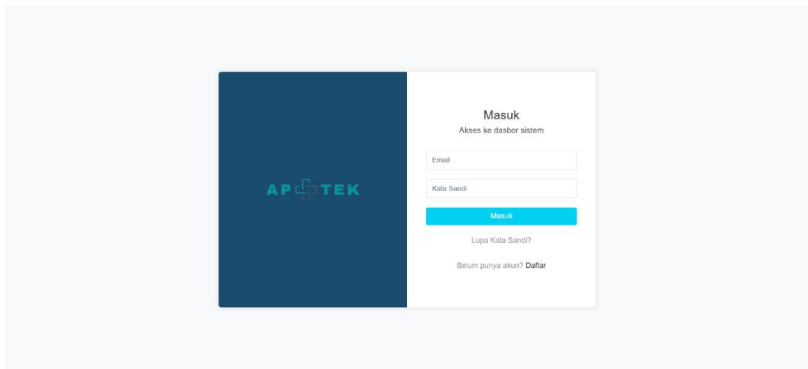
Gambar 7. Login
