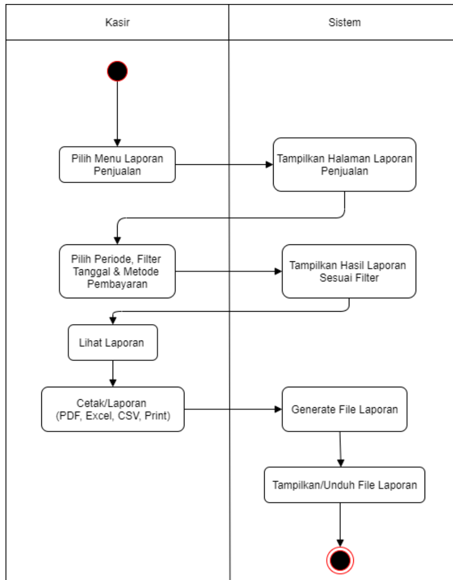
Gambar 6. Laporan
