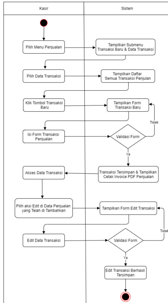
Gambar 4. Transaksi Penjualan
